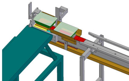
Produktvereinzlung 1 x 3 auf 1 x 1
