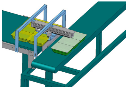
Produktvereinzlung 2 x 3 auf 1 x 3
